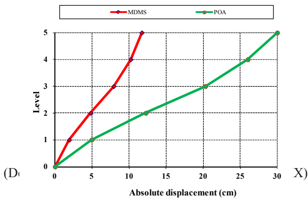
Figure 6: Absolute displacement for transversal direction YY (Déplacement absolu dans la direction transversal YY)
