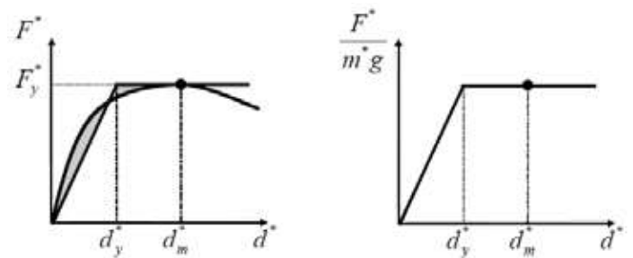
Figure 1 : Linearization of capacity curve (Linéarisation de la courbe de capacité)
