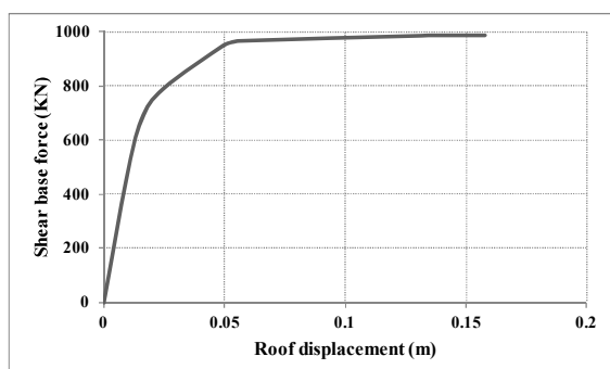
Figure 3: Capacity Curve for longitudinal direction XX (Courbe de capacité dans la direction longitudinale XX)
