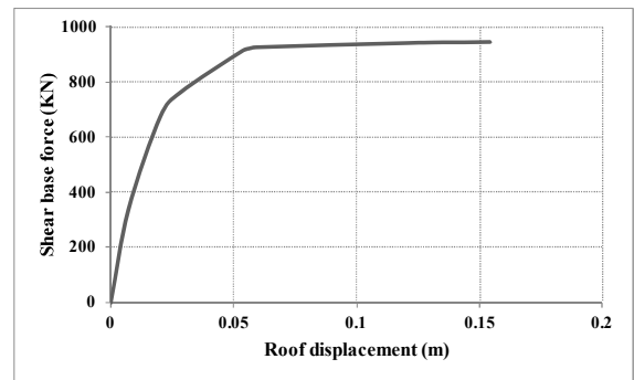
Figure 4: Capacity Curve for transversal direction YY (Courbe de capacité dans la direction longitudinale YY)
